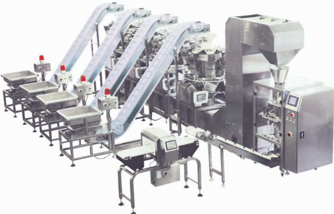
SBM – Verpackungsliniensystem mit Mehrkopfwaagen und Fördertechnik für unterschiedliche Beutelinhalte
